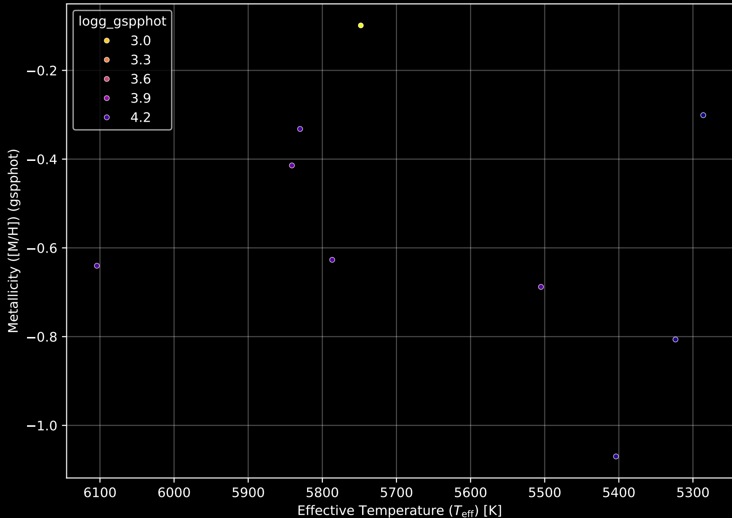
GALAH DR4 Field: [7375] Stellar Population Parameters (n= 9)
